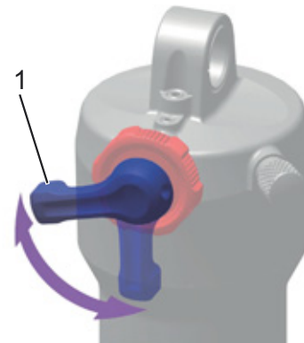
Rysunek 62: Ustawianie twardości tłumika dobicia za pomocą dźwigni (1) tylnego amortyzatora
